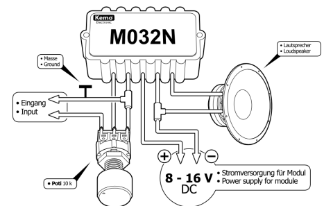
ANSCHLUSSPLAN | CONNECTION PLAN
