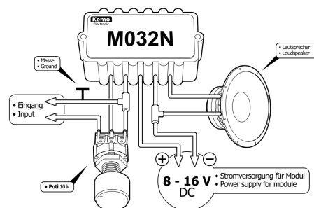
ANSCHLUSSPLAN | CONNECTION PLAN
